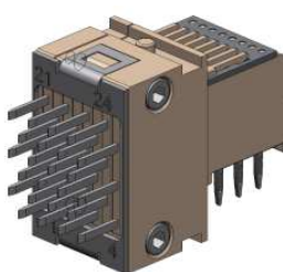
Blade side
