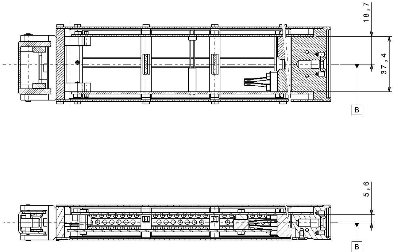
Picture 11 : section TYCO blade
