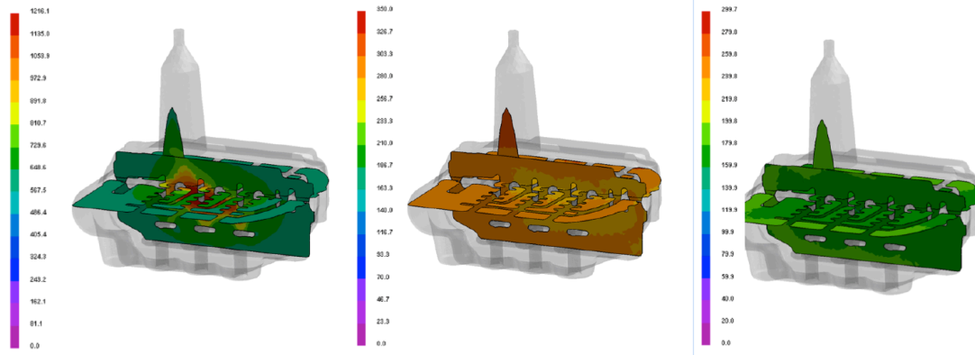
HARDNESS (Brinell)
