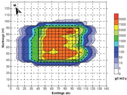
◆图5. 鱼排向沉积物输出的有机碳的模拟分布。
