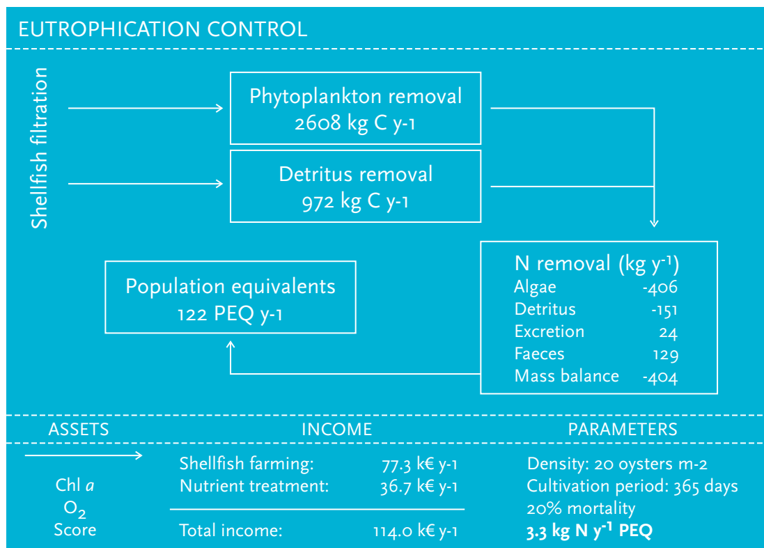
▲ 图6. 利用FARM模型计算的桑沟湾牡蛎养殖区物质输入/输出概况。
