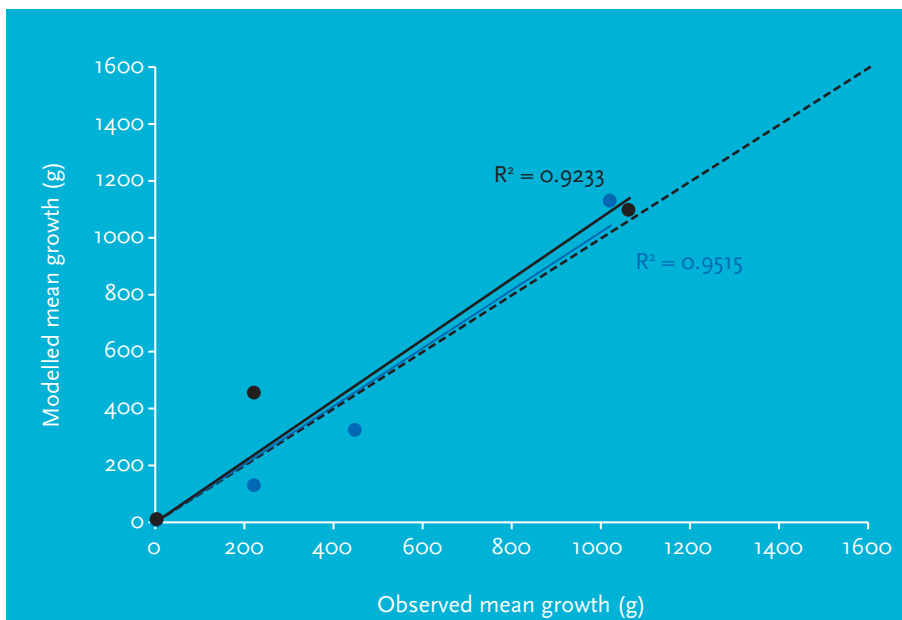
图3. 黄墩港示范点鲈鱼生长的TGC模型计算结果与观测值比较。
