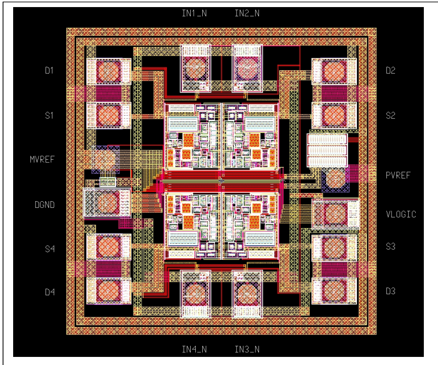
Fig. 5: ASIC A1 – Layout
